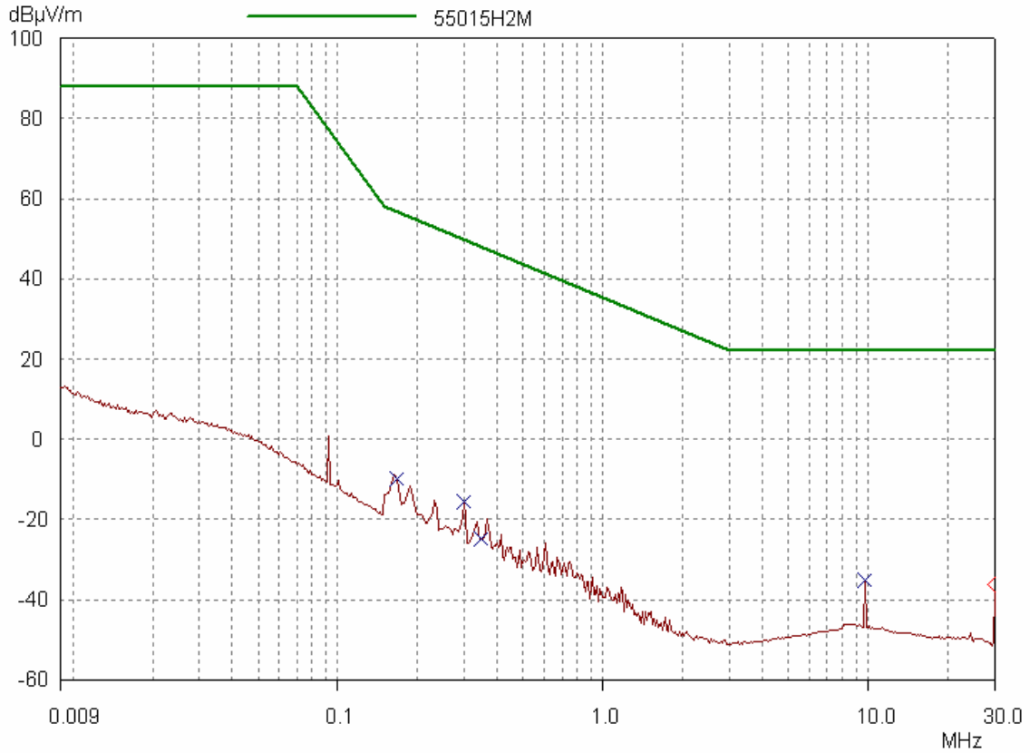
Plot 2e Q117RM1Z
